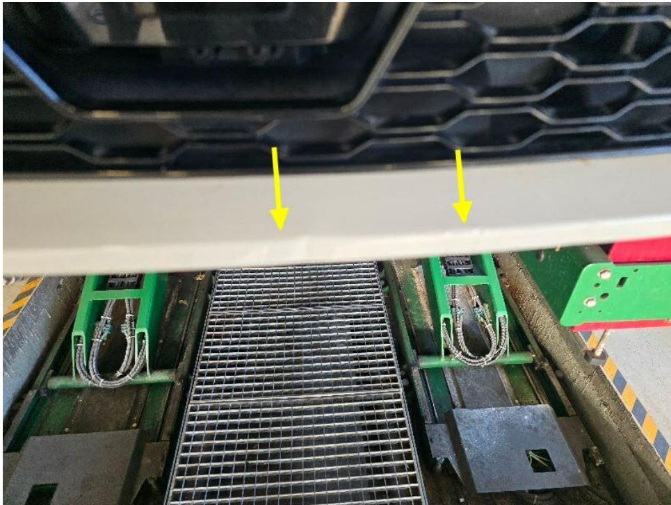
Bild 17 : Stoßfänger vorne, mehrfach eingedellt, instandsetzen und lackieren mit Lackaufbau
