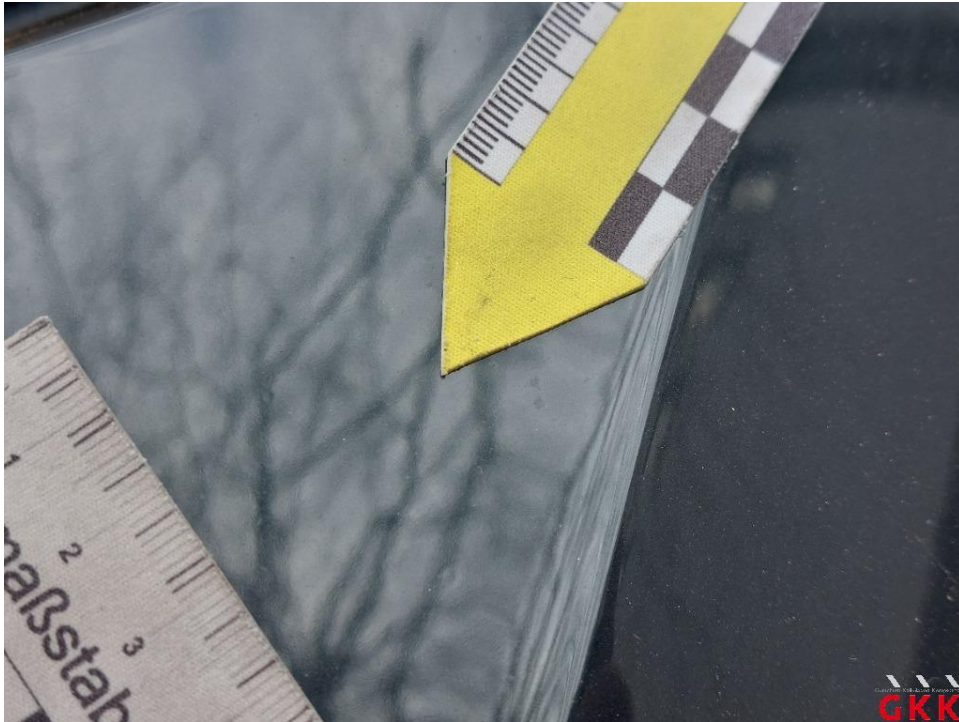
Bild 31. Motorhaube, Reparaturmangel, lackieren
