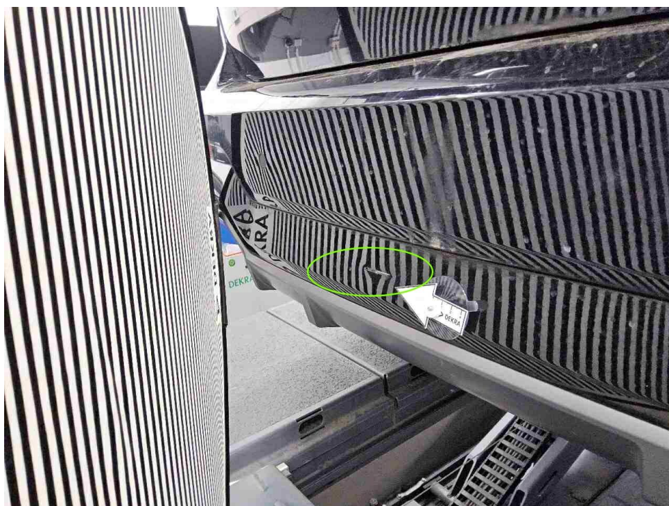
Bild 34 : Stoßfänger hinten unterhalb verkratzt und deformiert
