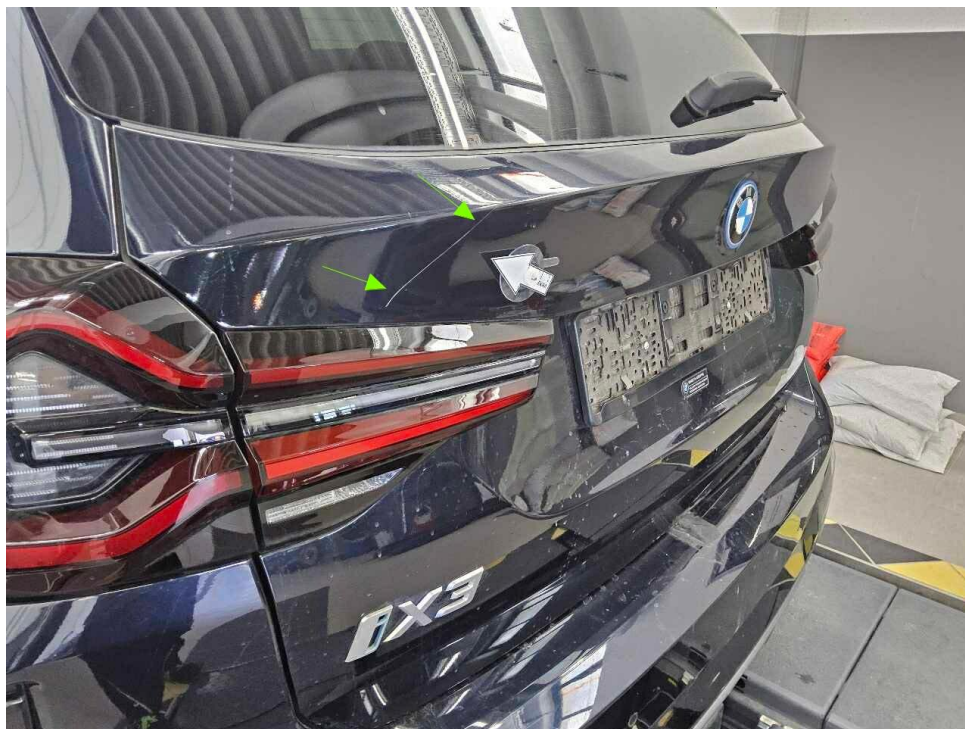
Bild 23 : Heckklappe Lackierung oberhalb, zerkratzt, lackieren mit Lackaufbau
