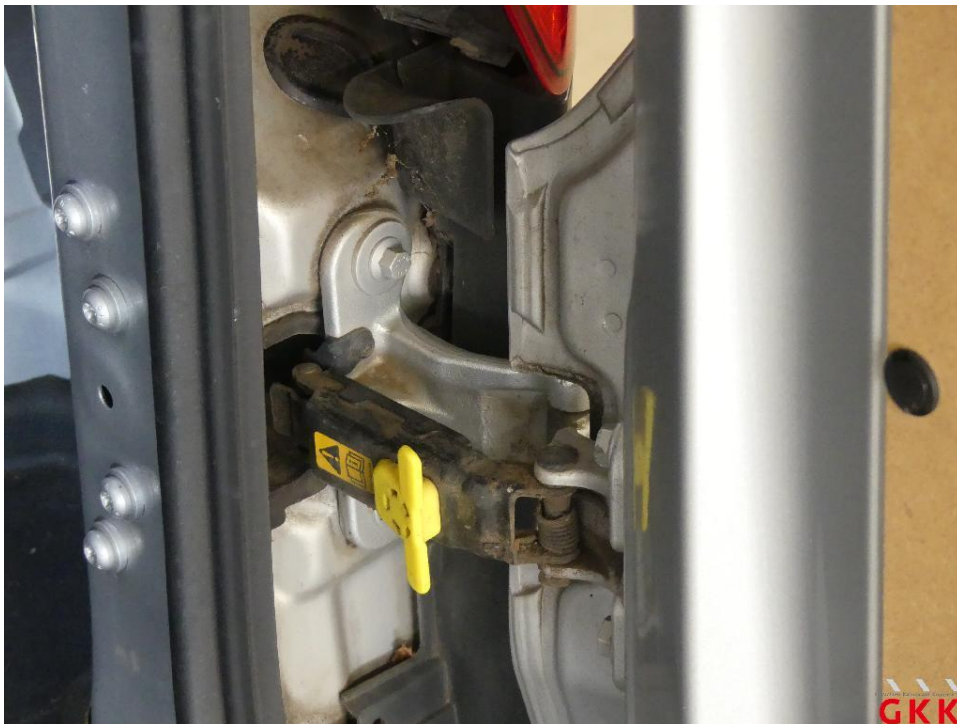
Bild 22 Hecktür rechts, Scharnier -unten-, schwergängig, instand setzen
