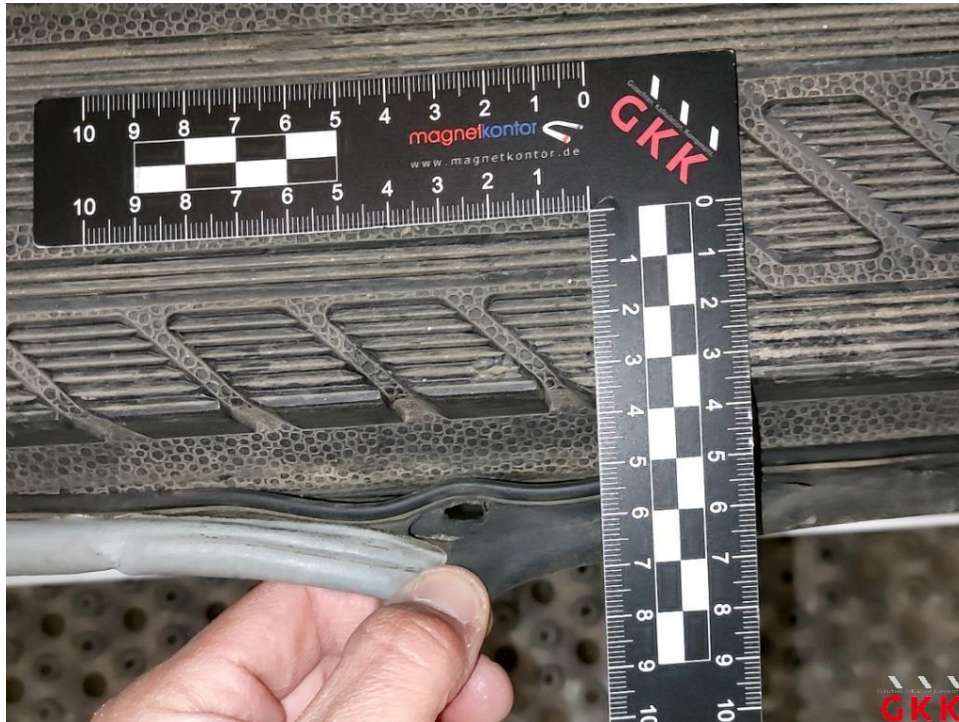
Bild 19 Schiebetür rechts, Dichtung -Einstieg-, beschädigt, ersetzen
