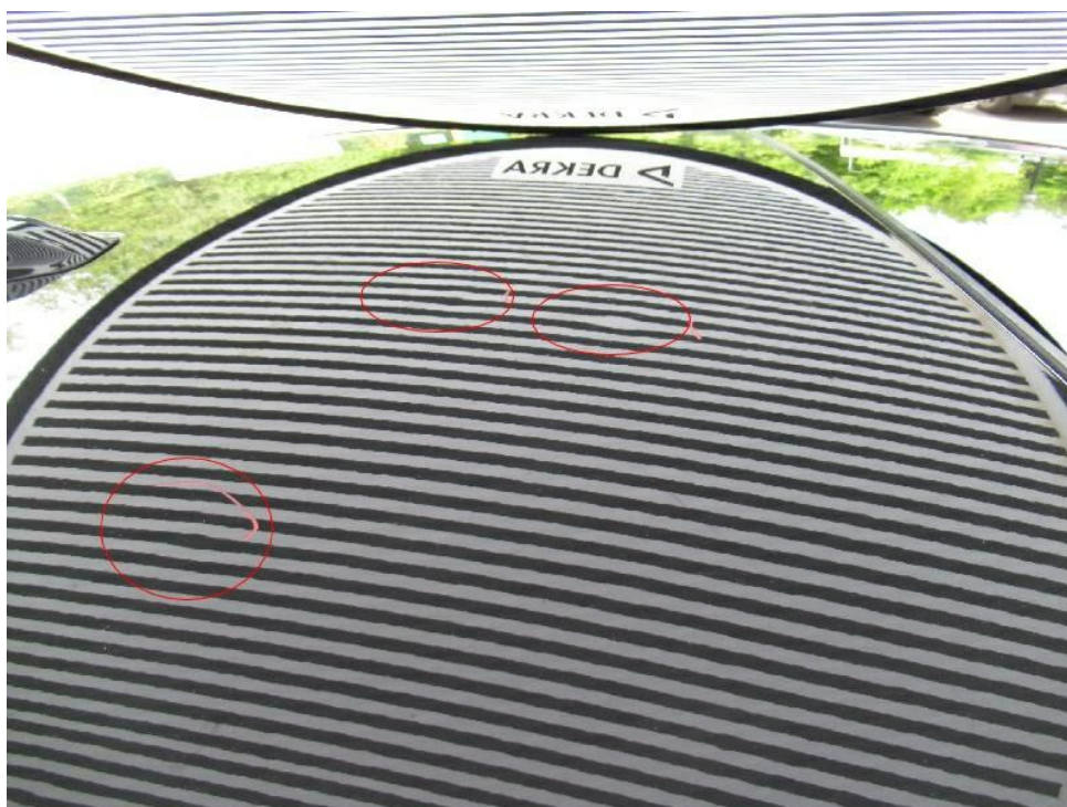
Bild 21 : Hagel-Umweltschaden an Dach und Heckdeckel
