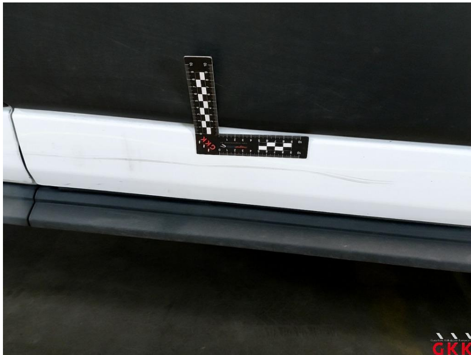
Bild 30 Tür vorne rechts, korrodiert, instand setzen - lackieren
