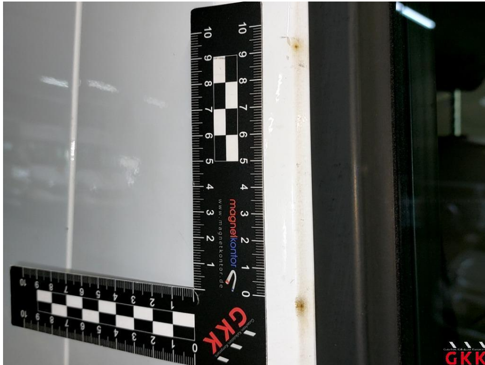
Bild 29 Tür vorne rechts, korrodiert, instand setzen - lackieren
