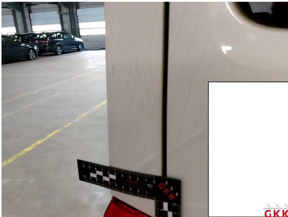
Bild 38 D- Säule links, beschädigt, Smartrepair
