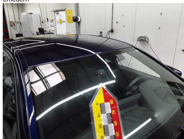
Beschädigung #5: Verglasung: Frontscheibe mit Spurhalteassistent - Steinschlag - erneuern
