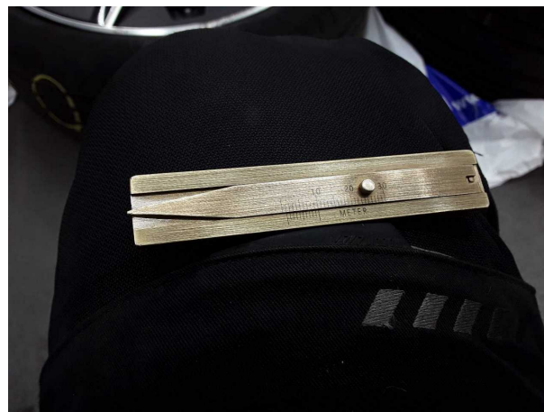
Beschädigung #4: 2.Radsatz: 2 Reifen - verschlissen - erneuern
