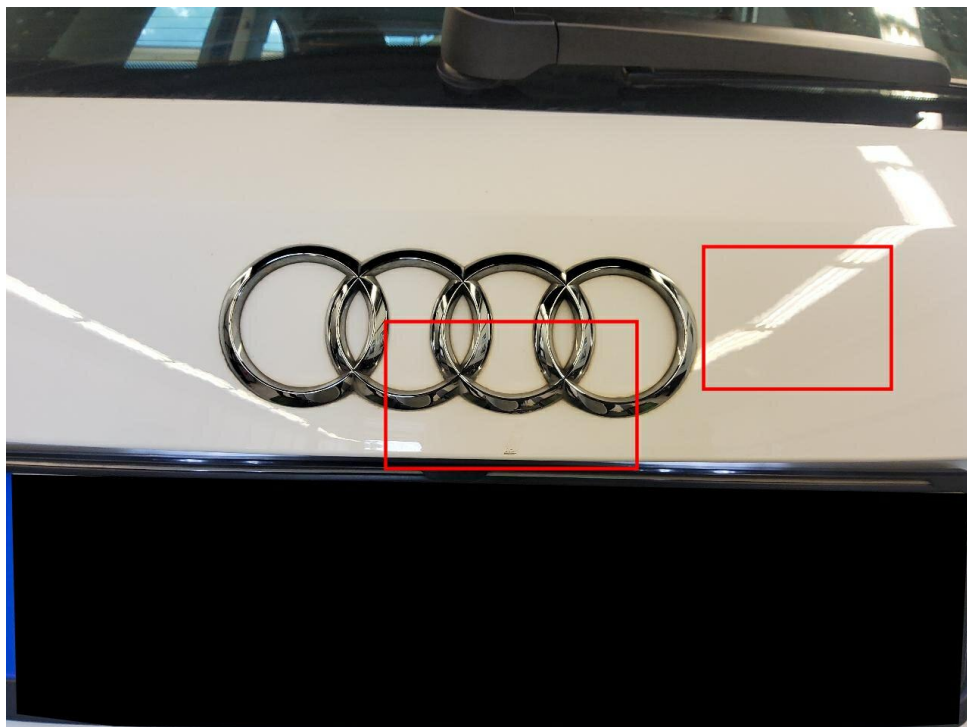
Bild 28 : Heckklappe, mehrfach eingedellt, instandsetzen und lackieren mit Lackaufbau
